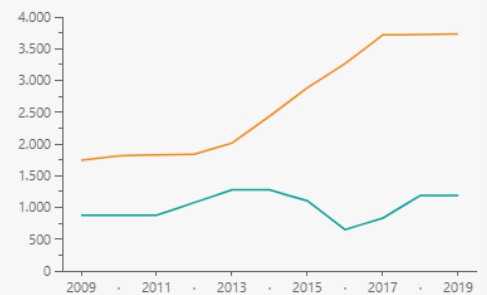
Potencia Instalada por Fuente (MW)
